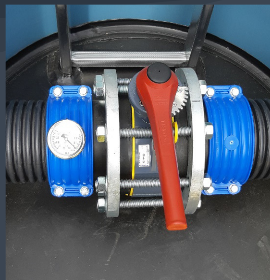
Conexión tubo corrugado MEGAPIPE SN16 – tubo liso PE100
